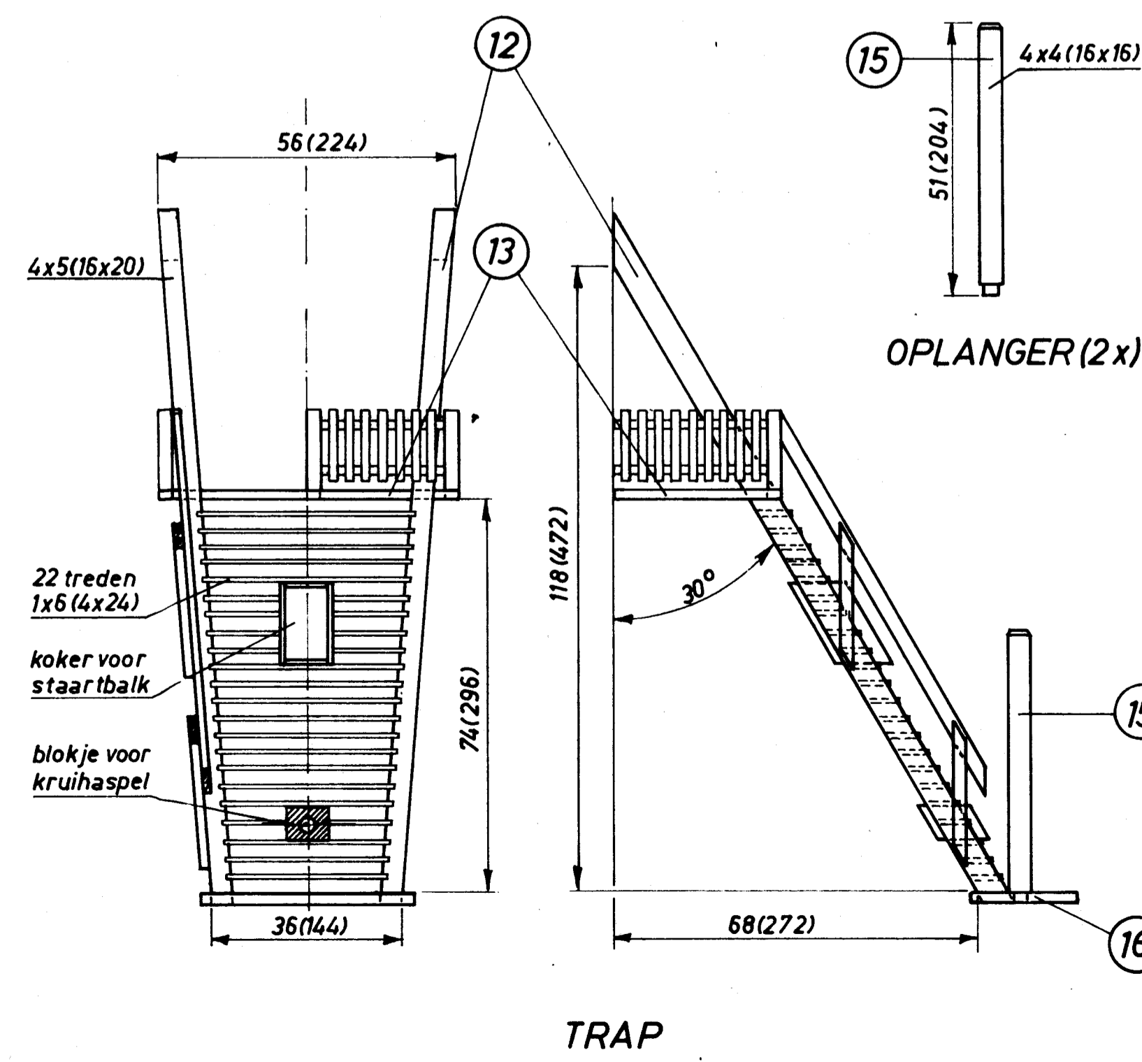
ZIJ-AANZICHT
